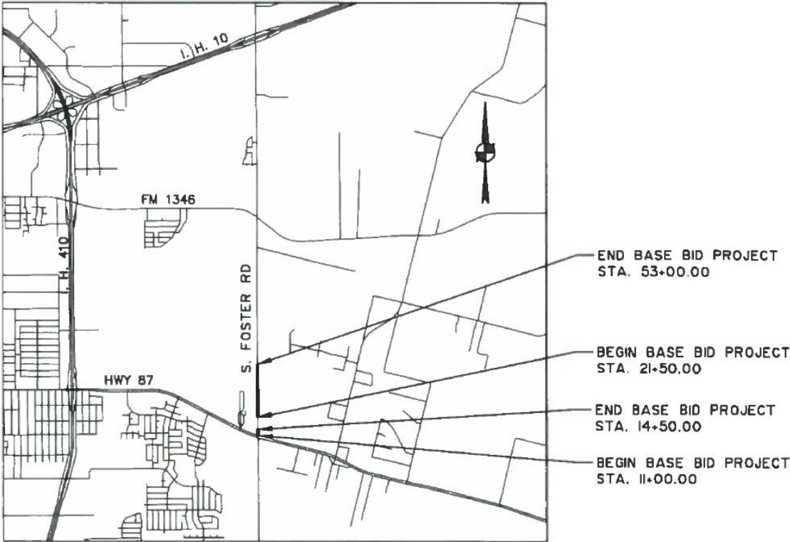
LOCATION MAP N.T.S. SAN ANTONIO, TEXAS
