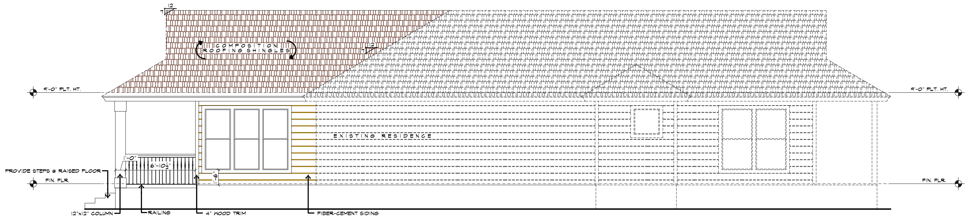
1 LEFT ELEVATION SCALE: 1/4"=1'-0"
