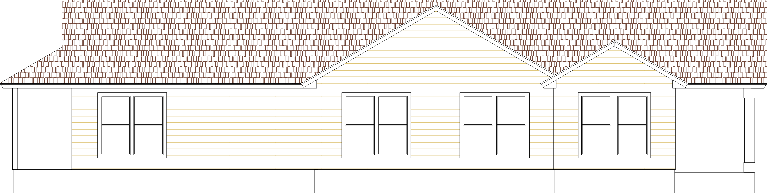
1 RIGHT ELEVATION SCALE: 1/4"=1'-0"
