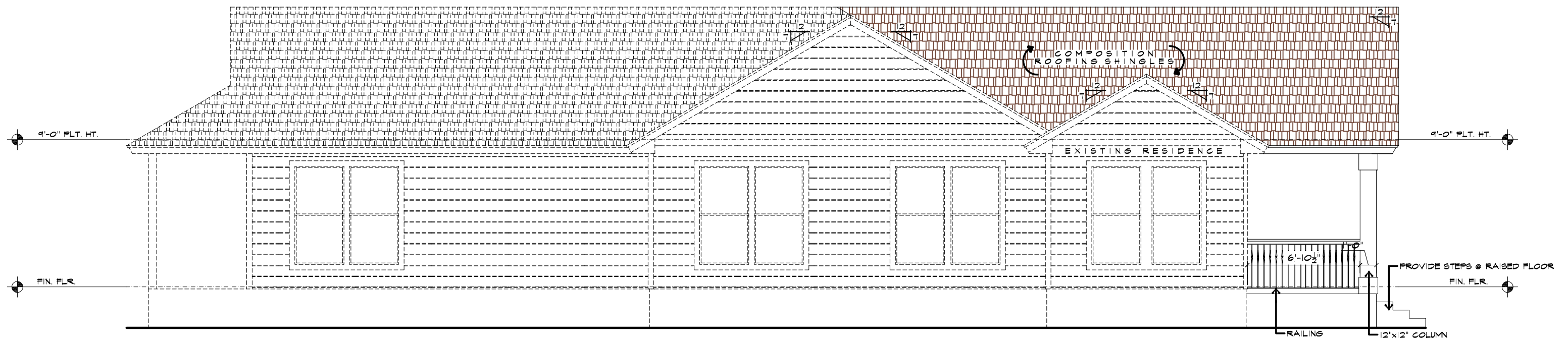
1 RIGHT ELEVATION SCALE: 1/4"=1'-0"
