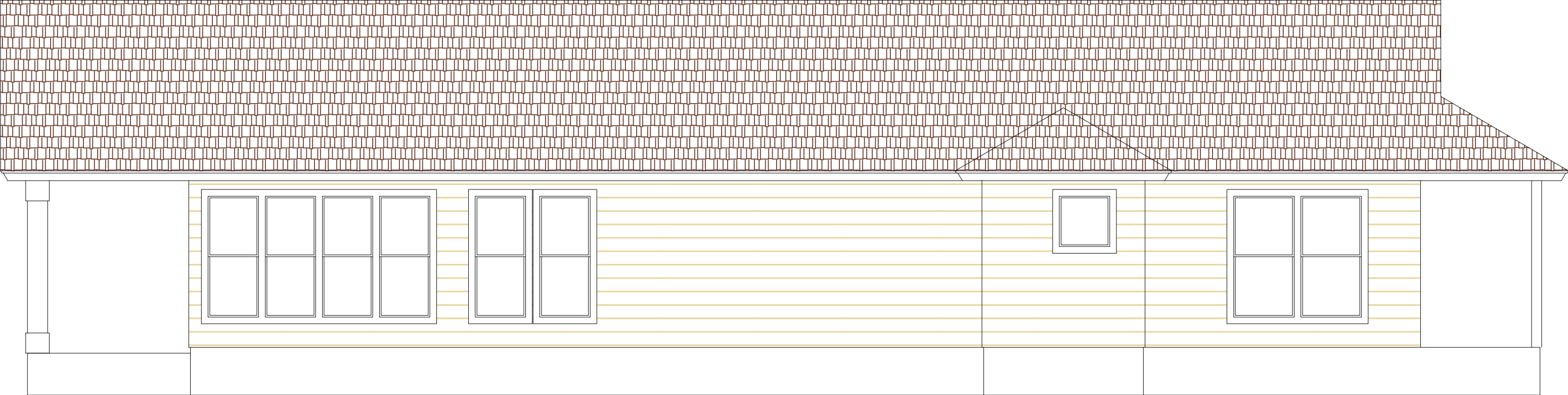
1 LEFT ELEVATION SCALE: 1/4"=1'-0"
