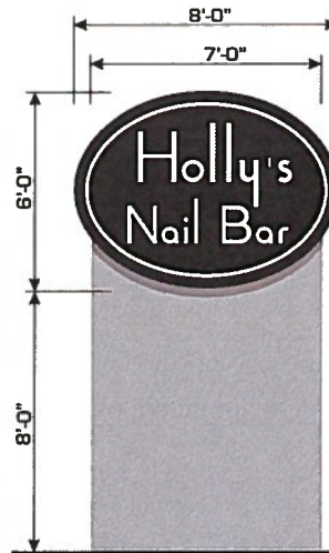
SCALE: 1/4" = 1'-0"
