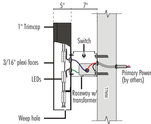
Typ. Side View - N.T.S.
