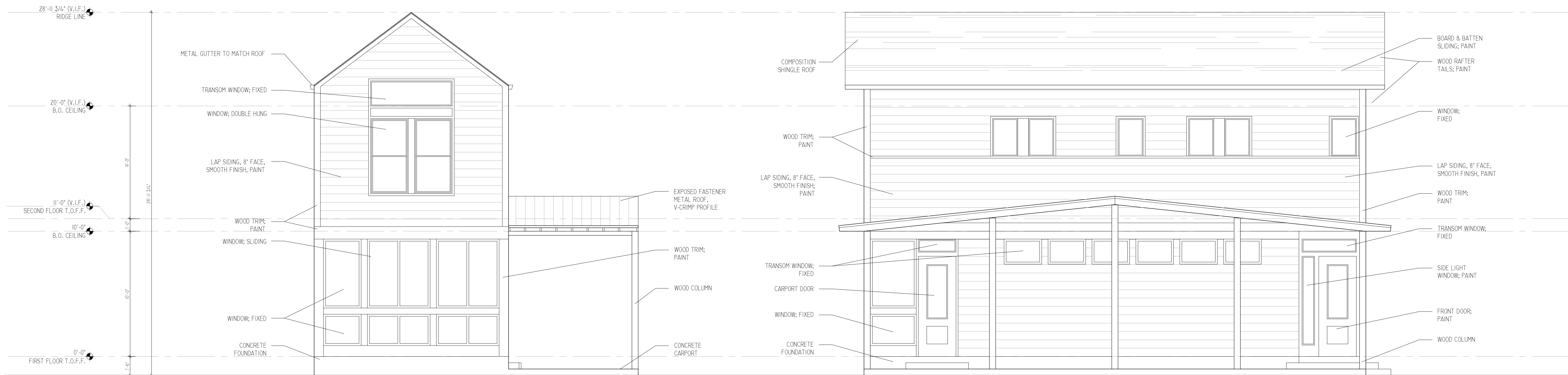
REAR ELEVATION - OPT A2 SCALE: 3/8" = 1'-0"
