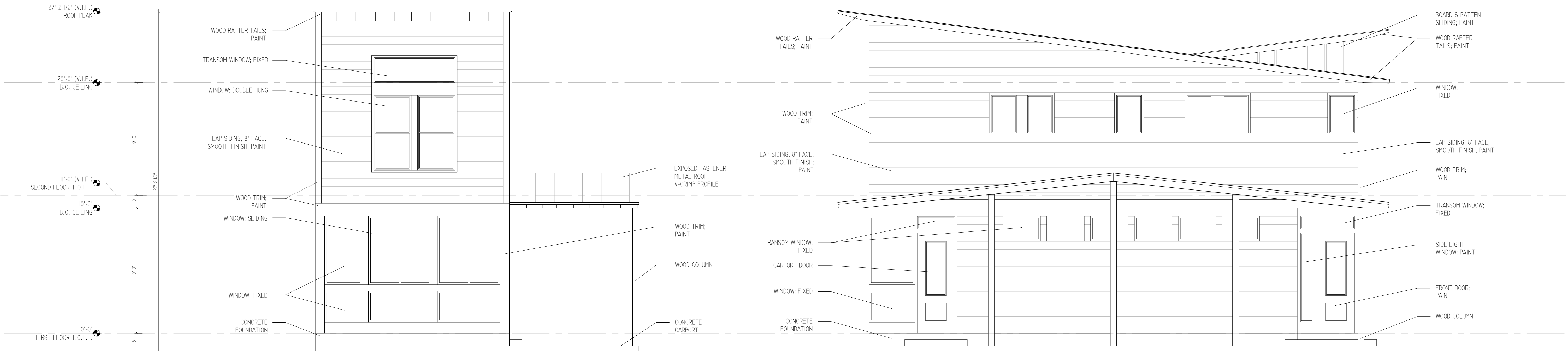
REAR ELEVATION - OPT AI SCALE: 3/8" = 1'-0"
