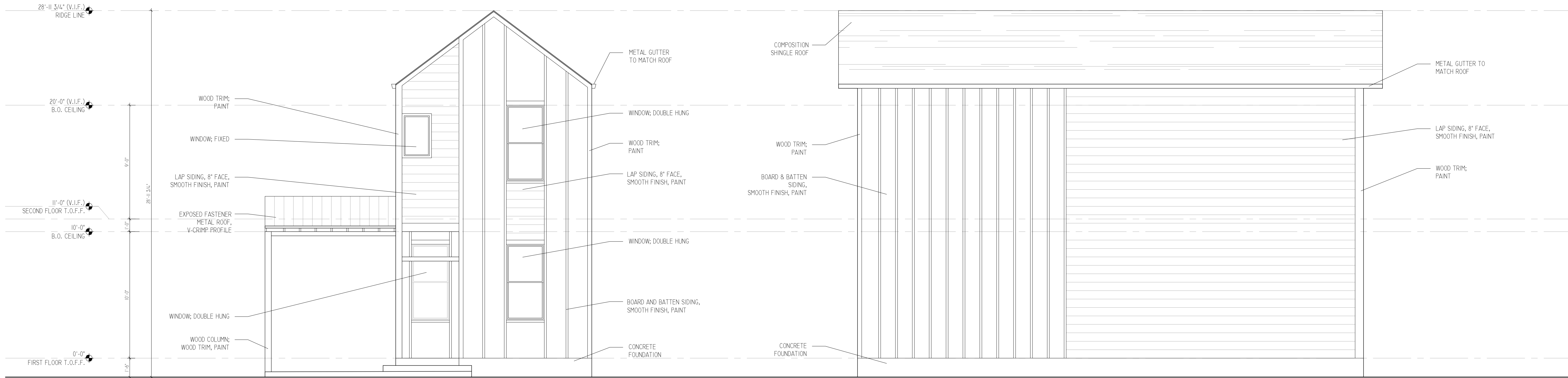
FRONT ELEVATION - OPT A2 SCALE: 3/8" = 1'-0"
